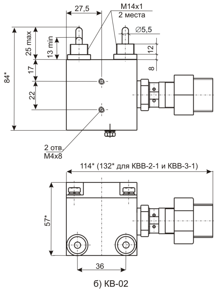
Рисунок А.1 – Габаритные, установочные и присоединительные размеры KB-01 и KB-02
