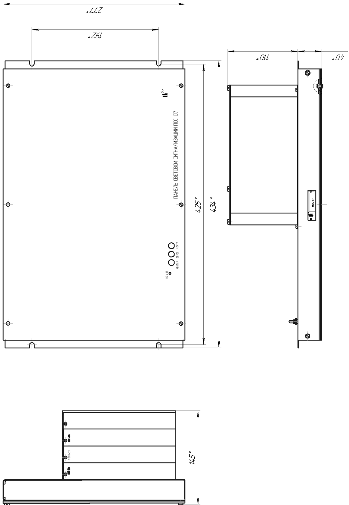
Рисунок Б.2 – Габаритные размеры ПСС-07-06, ПСС-07-07, ПСС-07-12(в исполнении ПСС-07-12 каркас с модулями ввода-вывода отсутствует)
