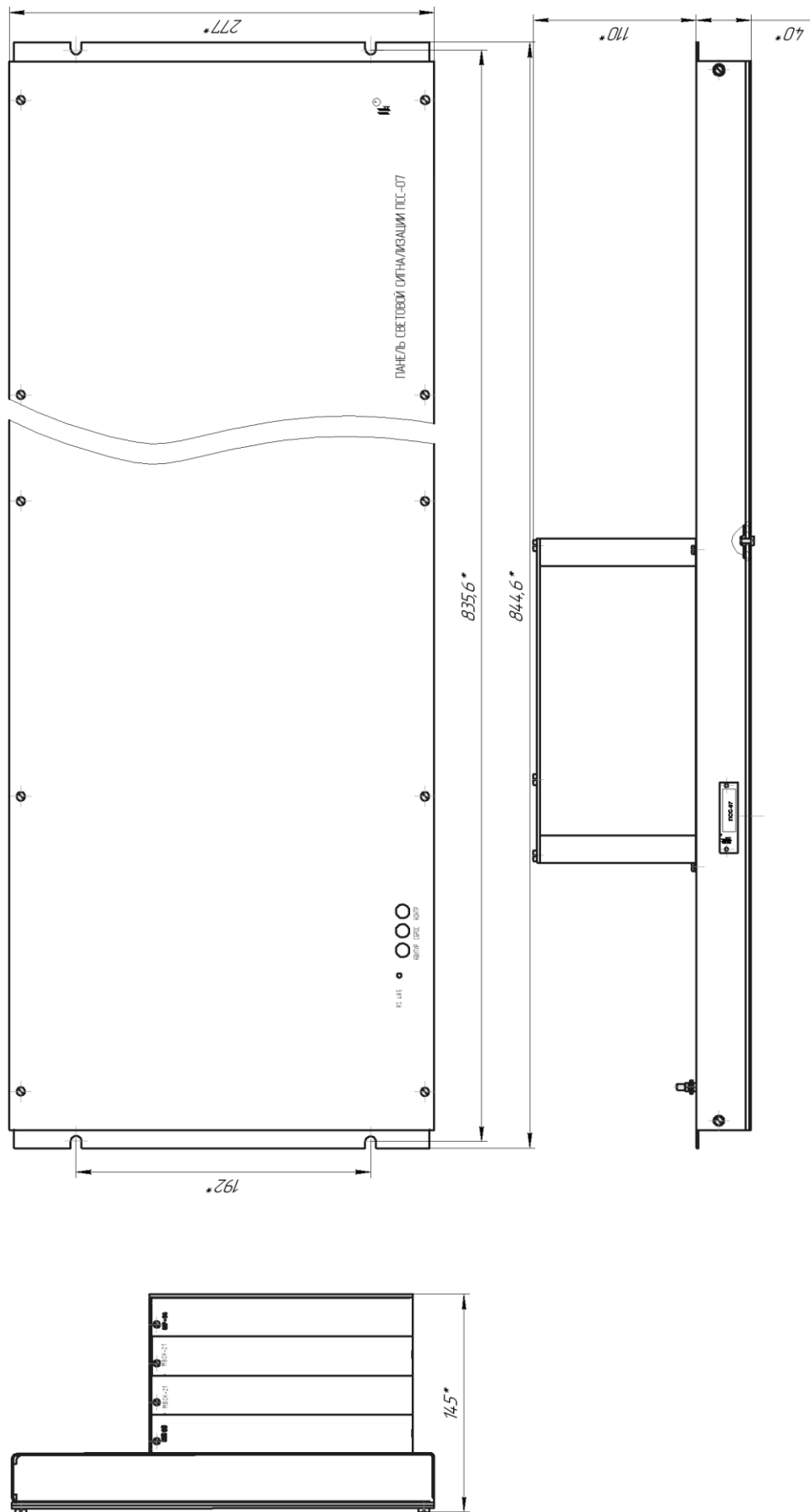
Рисунок Б.4 – Габаритные размеры ПСС-07-09, ПСС-07-13
