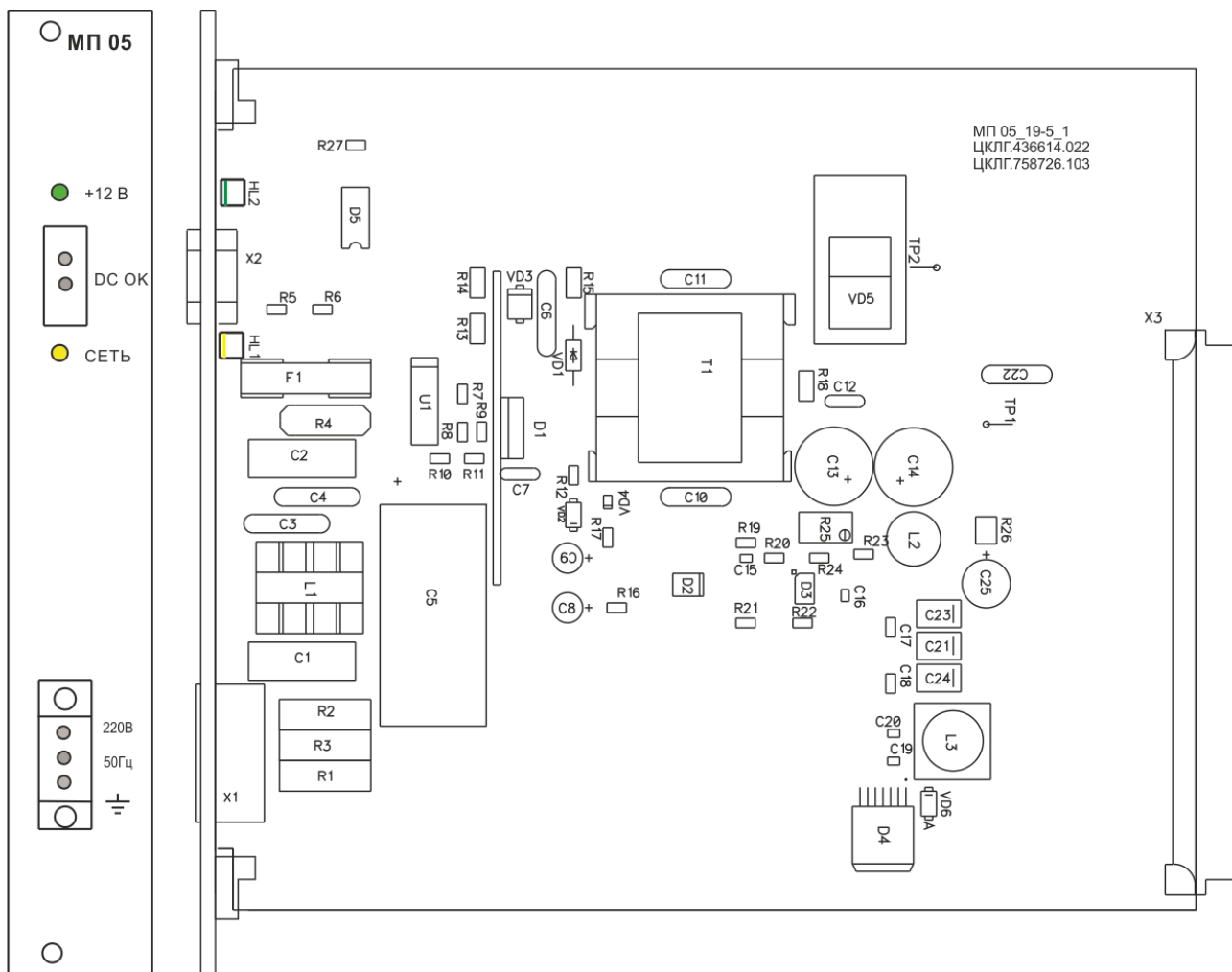
Рисунок 4.9 – Внешний вид печатной платы модуля питания МП-05
