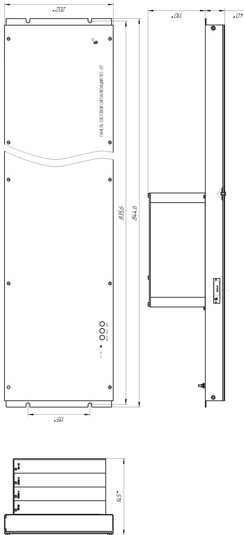
Рисунок Б.3 – Габаритные размеры ПСС-07-08, ПСС-07-11
