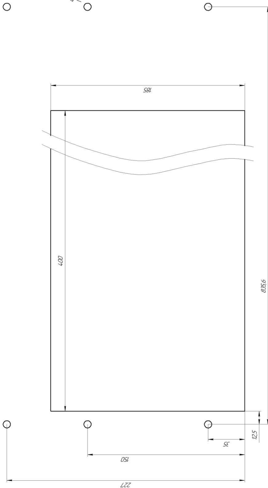
Рисунок Б.6 – Вырез в щите для исполнений ПСС-07 рисунок Б3, Б4
