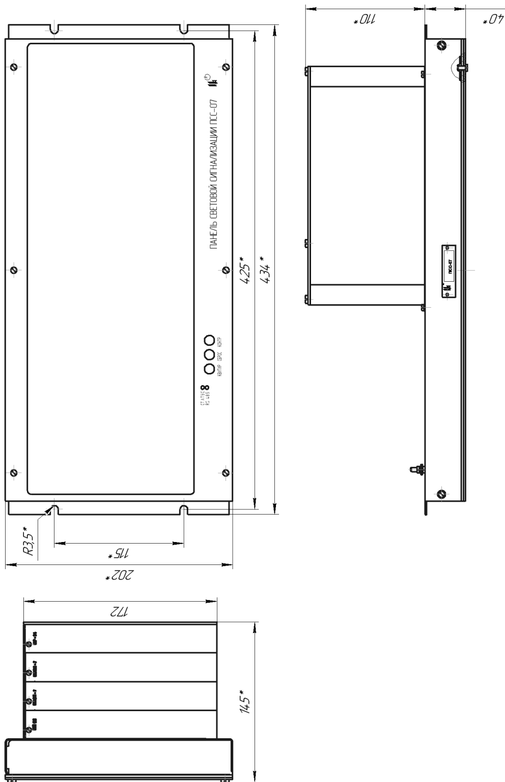
Рисунок Б.1 – Габаритные размеры ПСС-07, ПСС-07-01, ПСС-07-02, ПСС-07-04, ПСС-07-05, ПСС-07-10 (в исполнениях ПСС-07-01, ПСС-07-05 каркас с модулями ввода-вывода отсутствует)
