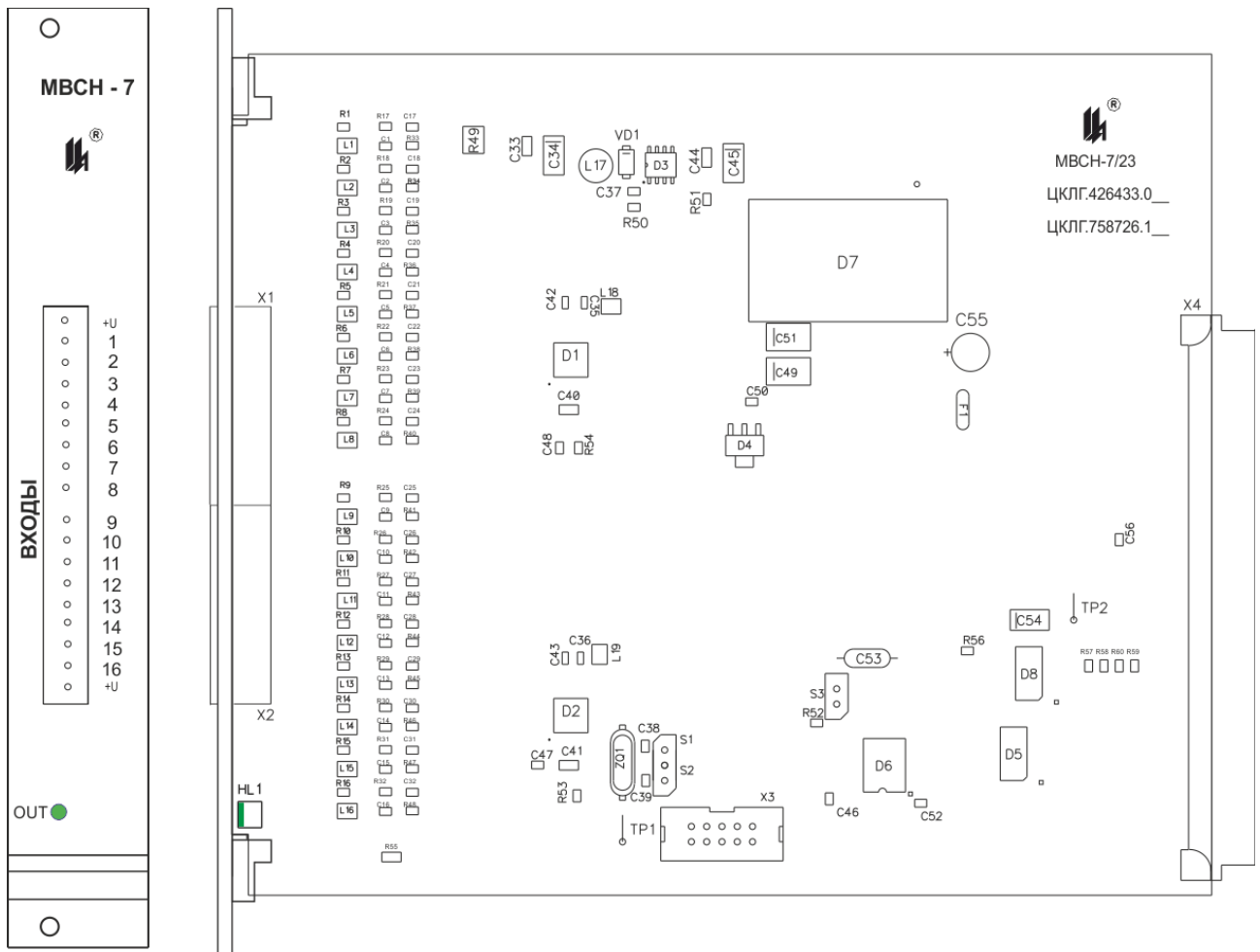
Рисунок 4.7 - Внешний вид платы модуля МВСН-7
